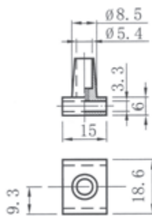
Στοπ συρταριών
